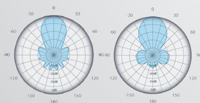
Diagrama de irradiação (horizontal) Azimute Elevação
